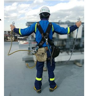
墜落制止用器具
